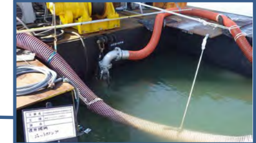
攪乱サンドポンプ用3t電動ウインチ
