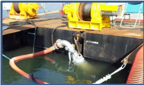
攪乱サンドポンプ用3t電動ウインチ
