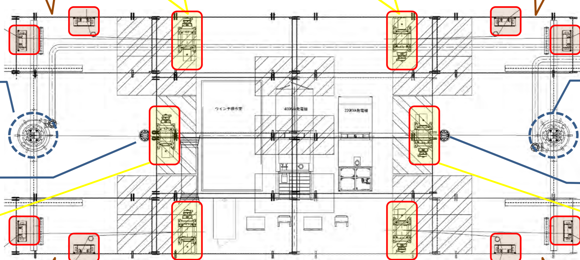
台船用3t電動ウインチ
